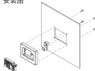
安装图
