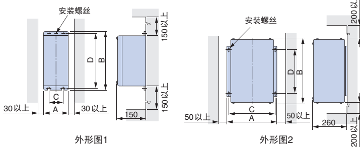
外形图1
