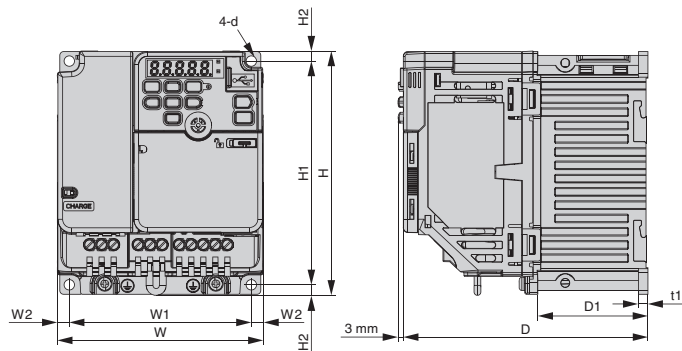
外形图 2
