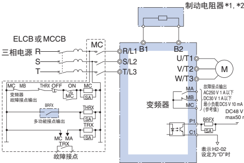
接线图A
