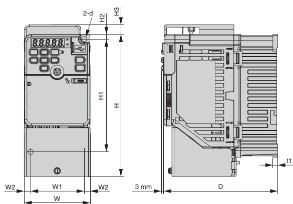
外形图 1
