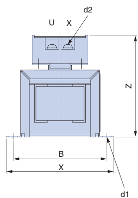
外形图1
