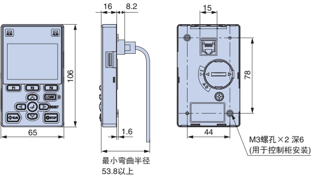
LCD操作器 外形尺寸 mm
