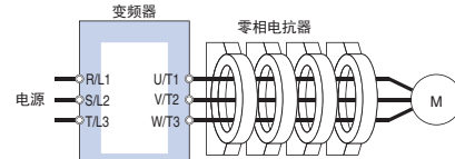
接线图b
