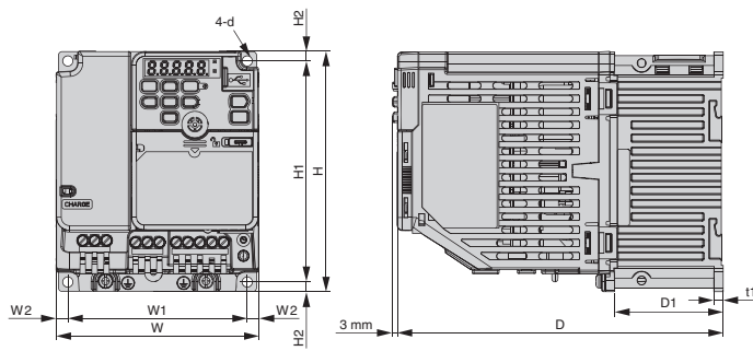
外形图 2
