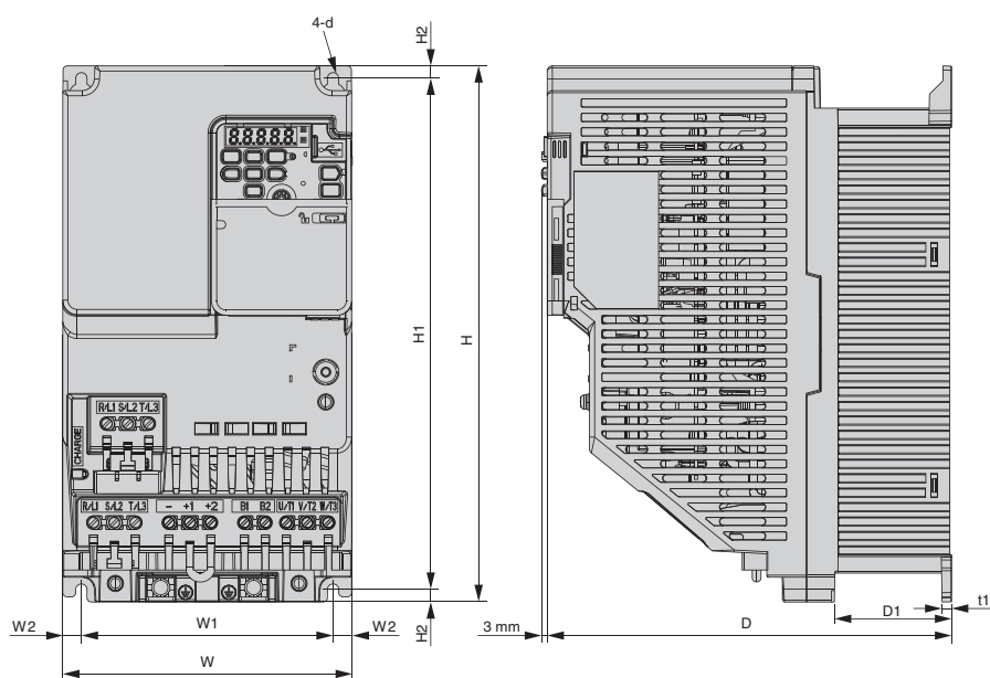
外形图 3
