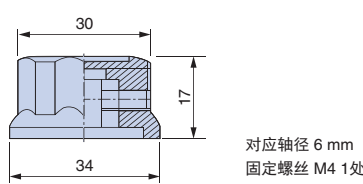
外形尺寸 mm
