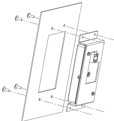
安装图(套件A时)
