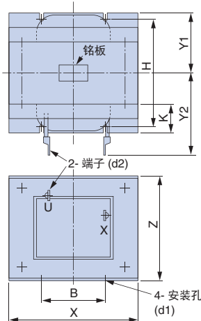
外形图 2
