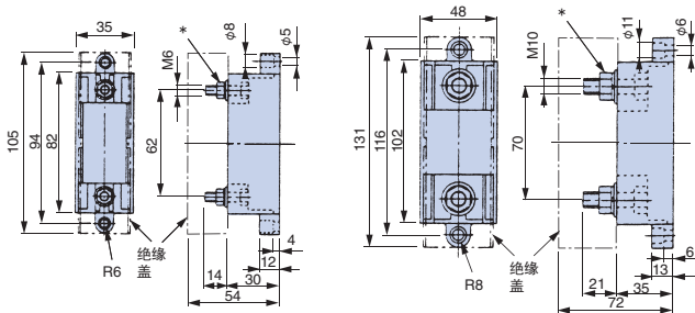
外形图1
