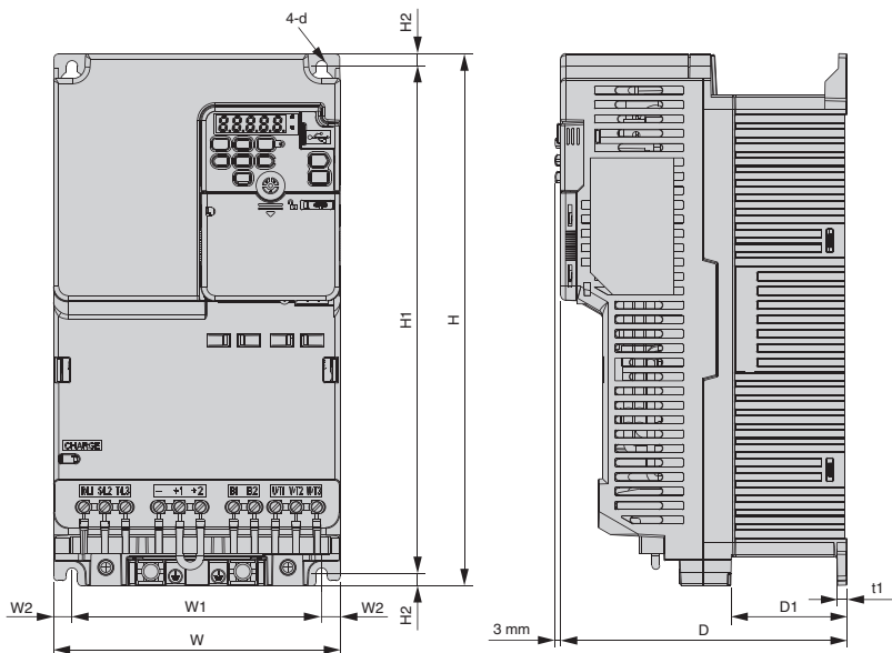
外形图 3
