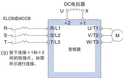
接线图
