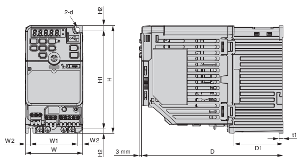
外形图 1
