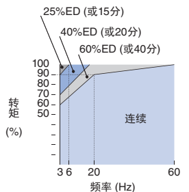
本公司标准电机的容许负载特性
