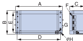
外形图2
