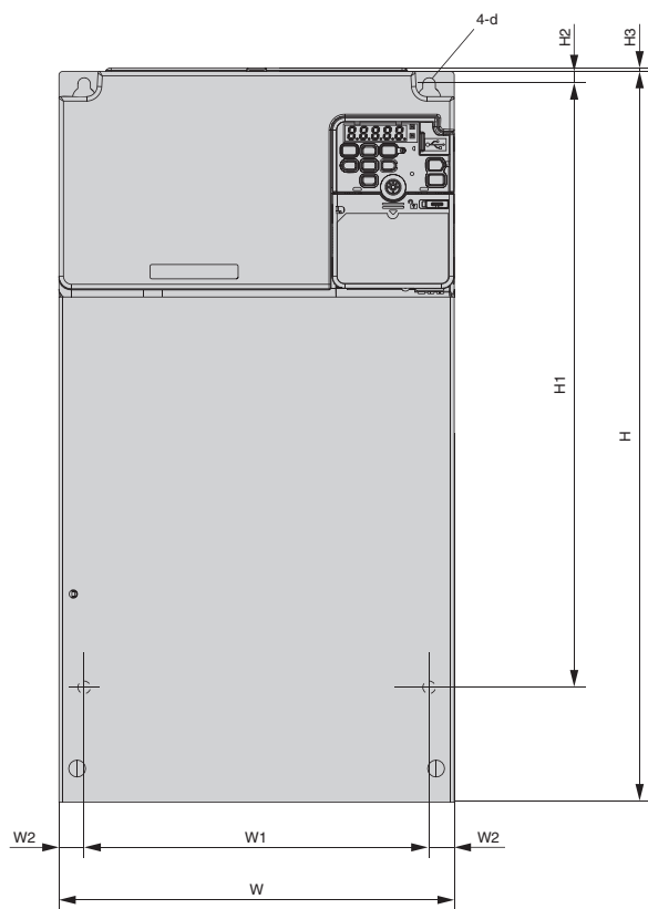
外形图 3
