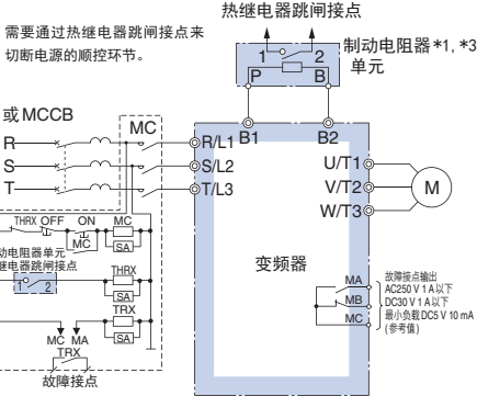
接线图B
