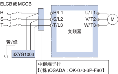
接线图
